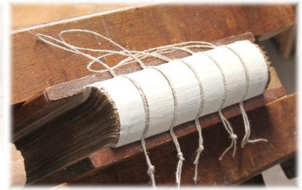
abgeleimter Buchblock ist gerundet, abgepresst in Handpresse, hinterklebt mit Büttenpapier
